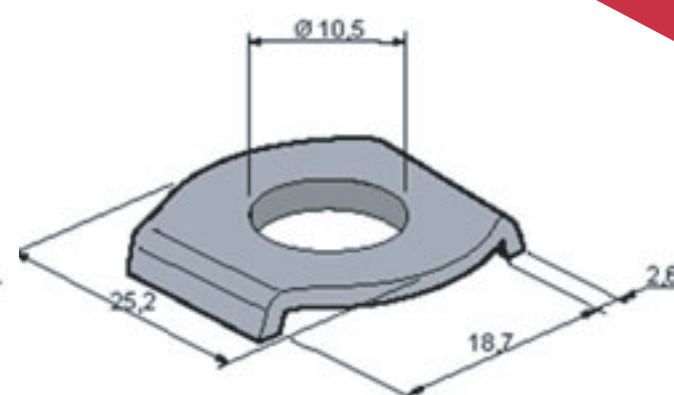
MODELO: ARD3/8
