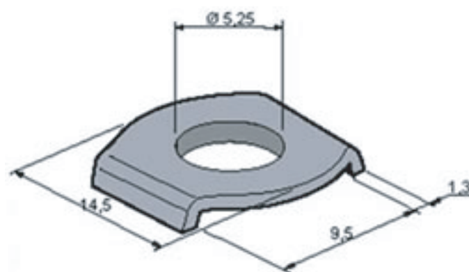
MODELO: ARD3/16
