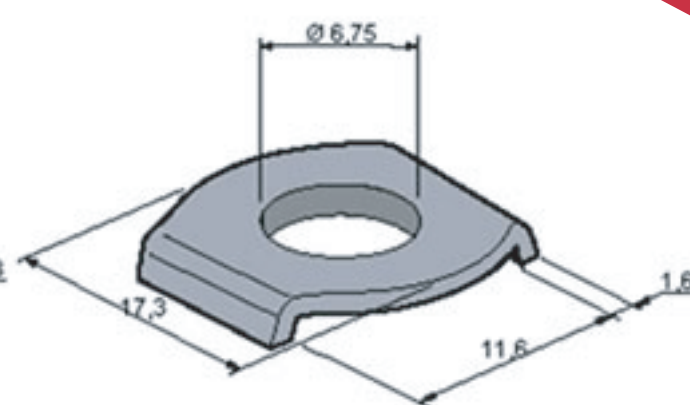
MODELO: ARD1/4
