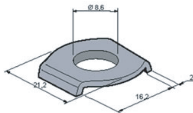
MODELO: ARD5/16
