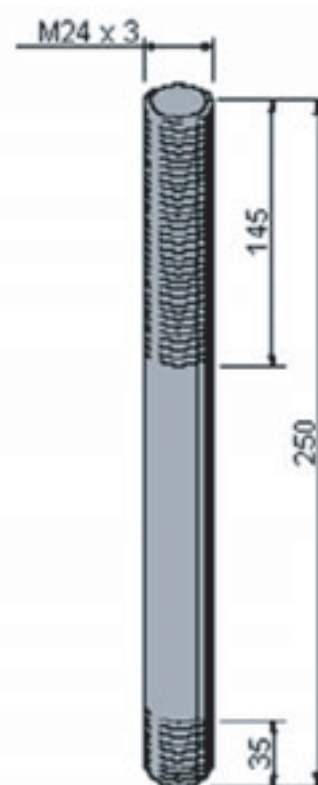
MODELO: M24 X 250 ARTICULO 602 - DIN 938
