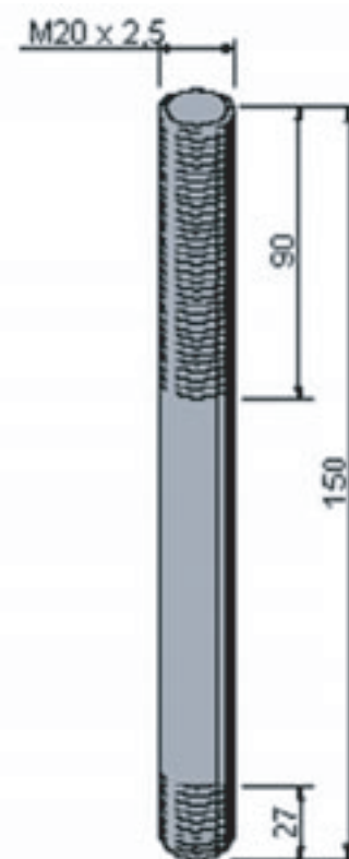
MODELO: M20 X 150 ARTICULO 602 - DIN 938
