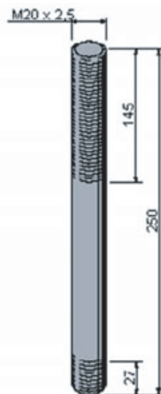
MODELO: M20 X 250 ARTICULO 602 - DIN 938
