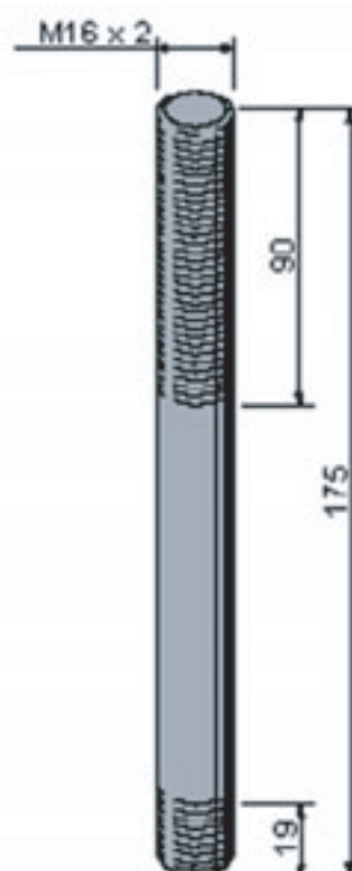
MODELO: M16 X 175 ARTICULO 602 - DIN 938
