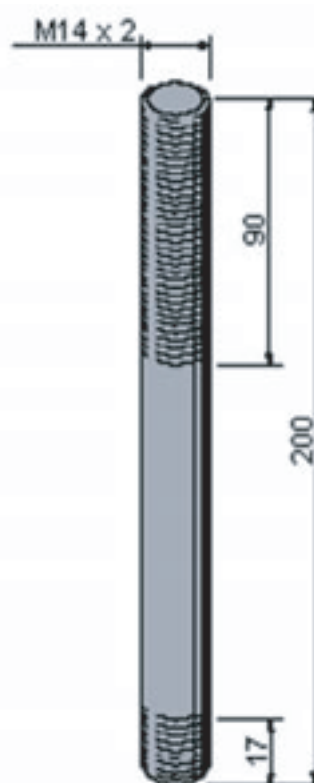
MODELO: M14 X 200 ARTICULO 602 - DIN 938
