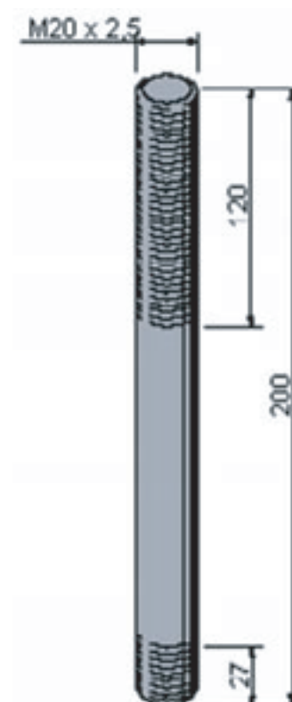
MODELO: M20 X 200 ARTICULO 602 - DIN 938
