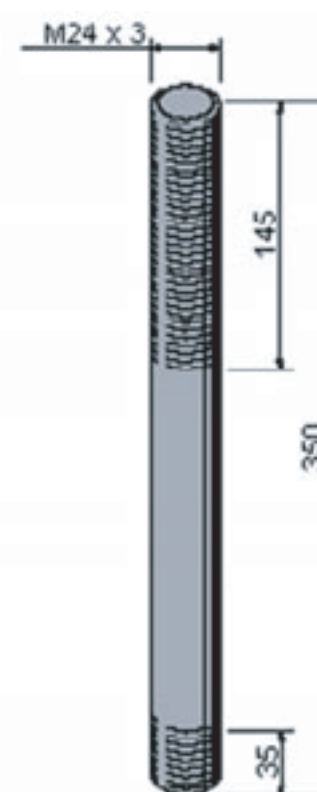
MODELO: M24 X 350 ARTICULO 602 - DIN 938
