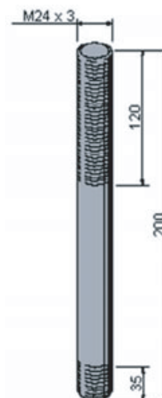
MODELO: M24 X 200 ARTICULO 602 - DIN 938
