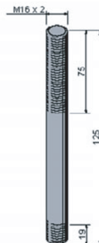
MODELO: M16 X 125 ARTICULO 602 - DIN 938
