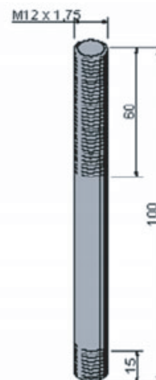
MODELO: M12 X 100 ARTICULO 602 - DIN 938
