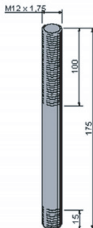
MODELO: M12 X 175 ARTICULO 602 - DIN 938
