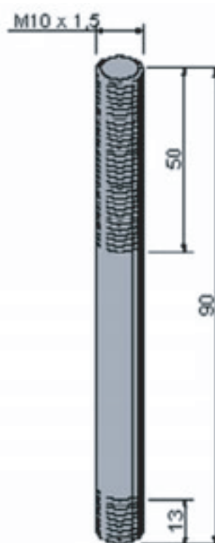
MODELO: M10 X 90 ARTICULO 602 - DIN 938
