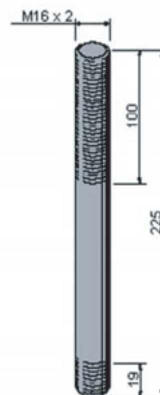
MODELO: M16 X 225 ARTICULO 602 - DIN 938
