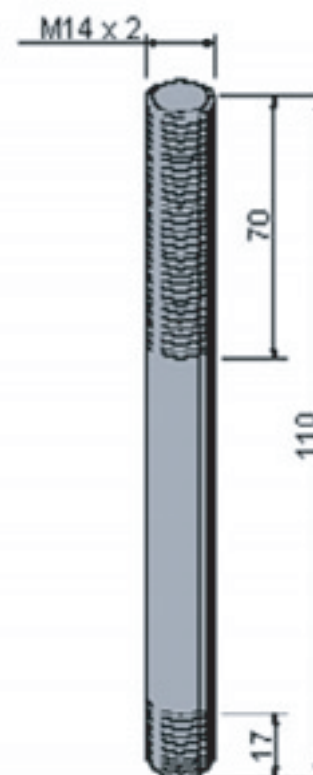
MODELO: M14 X 110 ARTICULO 602 - DIN 938
