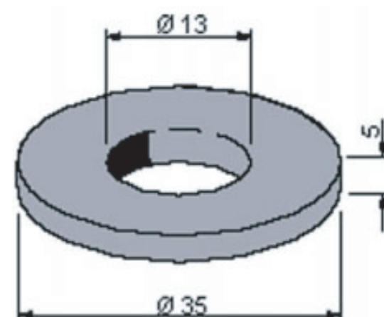
MODELO: D13 ARTICULO 604 - DIN 6340
