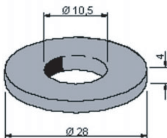
MODELO: D10.5 ARTICULO 604 - DIN 6340
